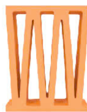
GẠCH W 260 MÃ SP: T42 - 19 %/m 2 KT: 260x200x60 (mm)
