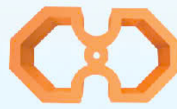
GẠCH CÁNH BƯỚM MÃ SP: T03 - 29 %/m 2 KT: 250x140x60 (mm)
